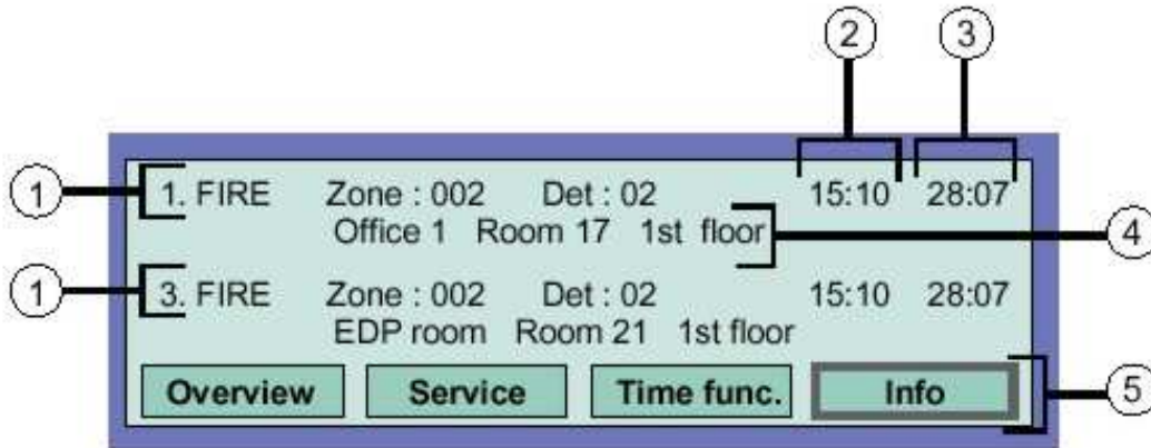
Slika 11. Primer prikaza požarnog alarma ( dodatni prikaz )
